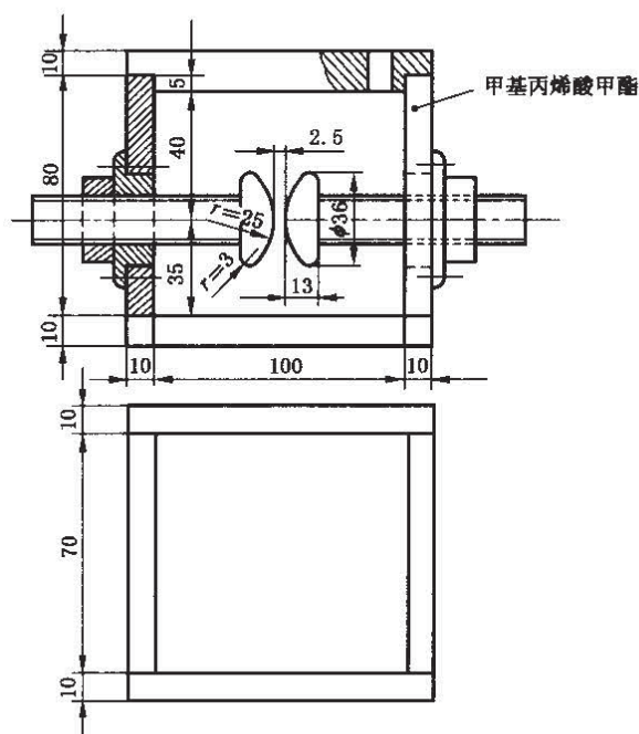
图 2 试样杯和球盖形电极示意图
