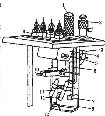
图 B1 继电器的芯子结构
