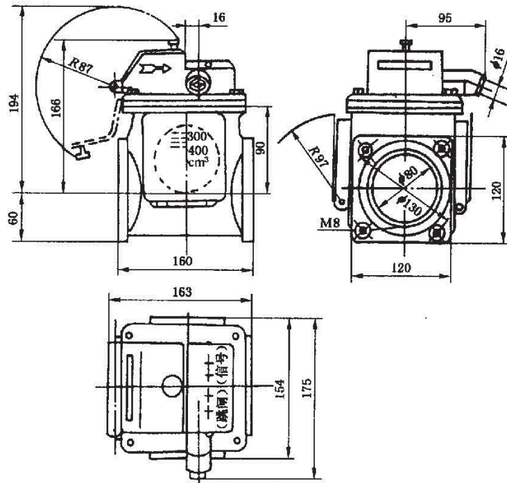
图 B2 继电器外形图
