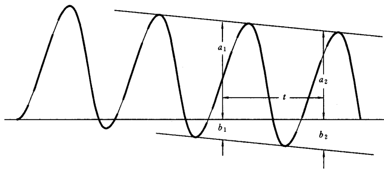
a TPZ 级电流互感器一次时间常数的测量
