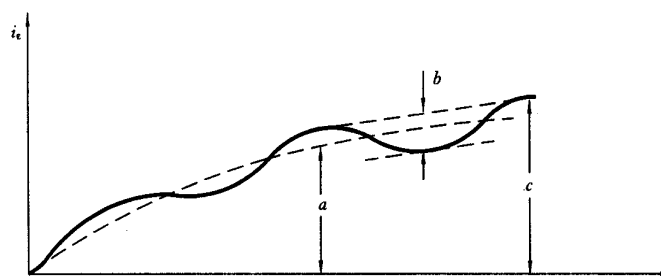
a TPZ 级电流互感器一次时间常数的测量
