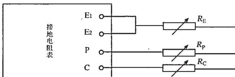
图2 R_x \leq 10\Omega 时的原理接线图
