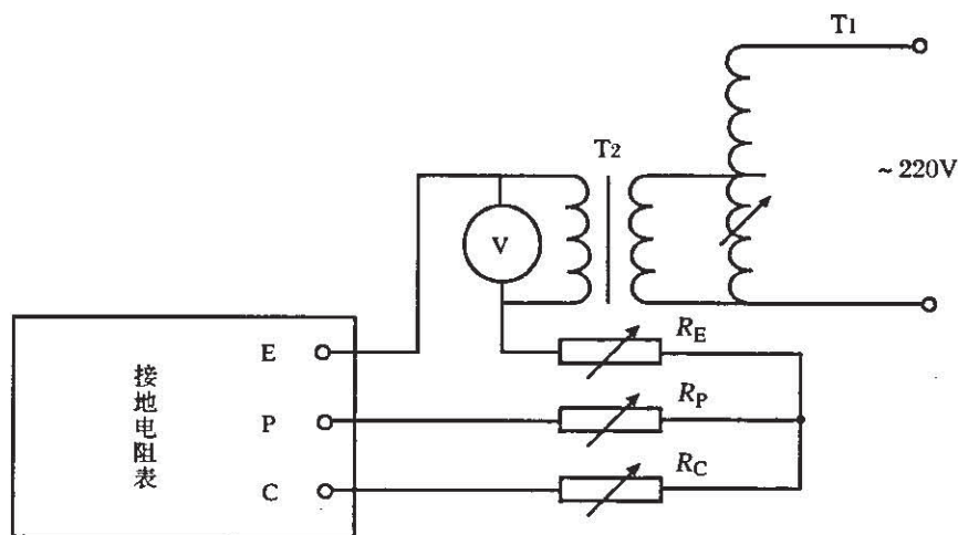
图3 地电压影响试验原理图
